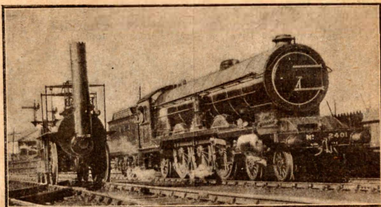
Et Aarhundredes Udvikling, klart belyst ved at stille Fortid og Nutid op ved Siden af hinanden. Billedet er taget paa Darlington Station ved Hundrekaarstidspunktet i 1925, hvor man har hentet det gamle »Locomotion« ud fra Museet og stillet det op ved Siden af et af de moderne Kæmpelokomotiver.
