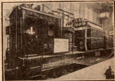
Transportabel elektrisk Transformator-Station paa de italienske Statsbaner. Hvis der indtræffer et Uheld med en af de faeste Transformatorstationer, bliver den transportable Station koblet til et Lokomotiv, og hurtigst muligt kørt til det paagældende Sted, saa den regelmæssige Drift kan genoptages.
